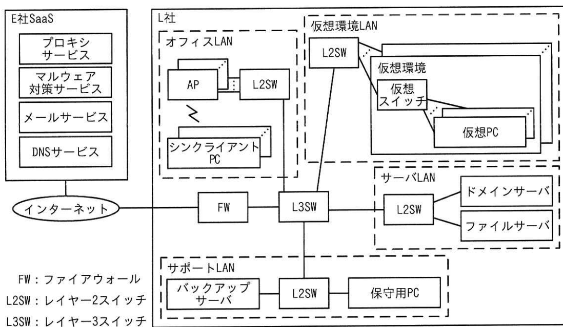
図1 L社のネットワーク構成（抜粋）
