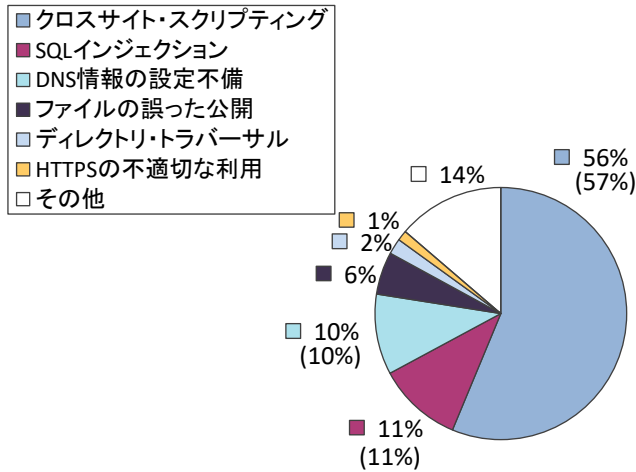
図2-15. 届出累計の脆弱性の種類別割合
