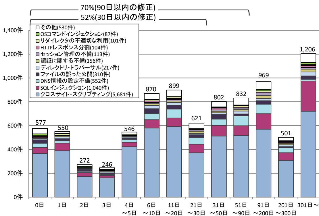
図2-20. ウェブサイトの修正に要した日数
