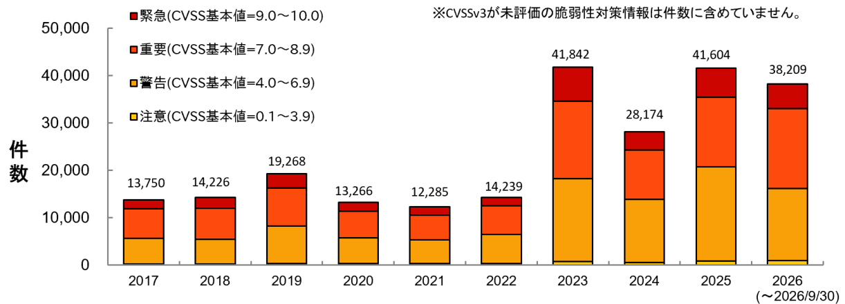
図 2-3. 脆弱性の深刻度別件数(CVSSv3) 過去 10 年分
