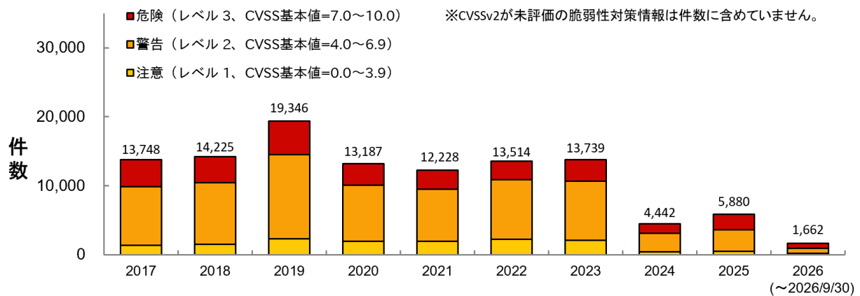
図 2-2. 脆弱性の深刻度別件数(CVSSv2) 過去 10 年分
