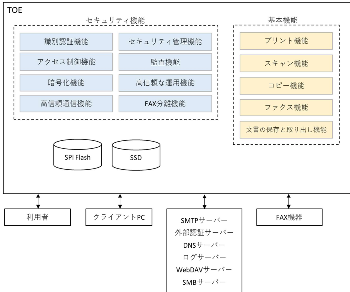
図 1-2 TOE の論理的範囲
