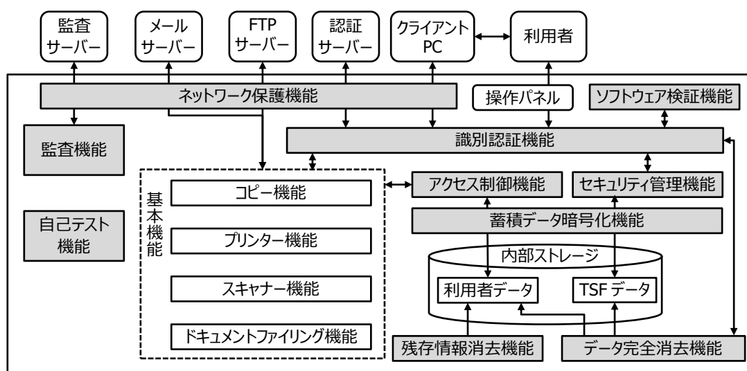
Figure 2: TOE の論理的構成
