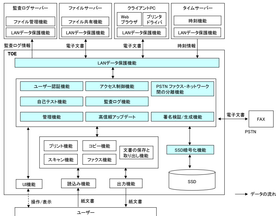
図 5-1 TOE の構成
