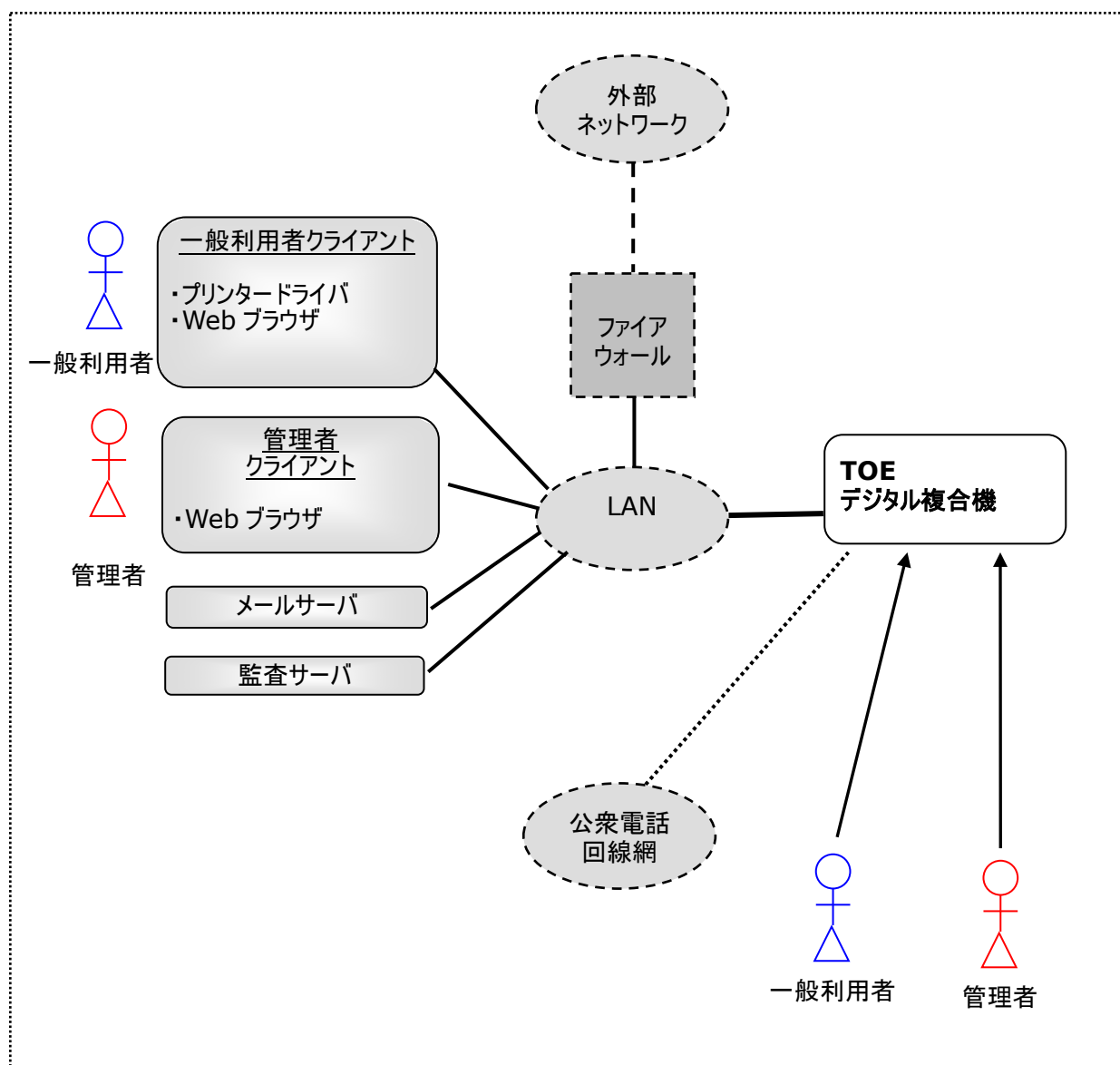
図 1 TOE の想定する運用環境
