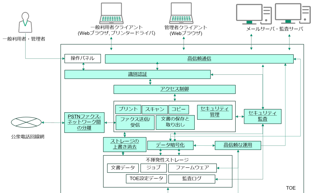
図 5-1 TOE の構成
