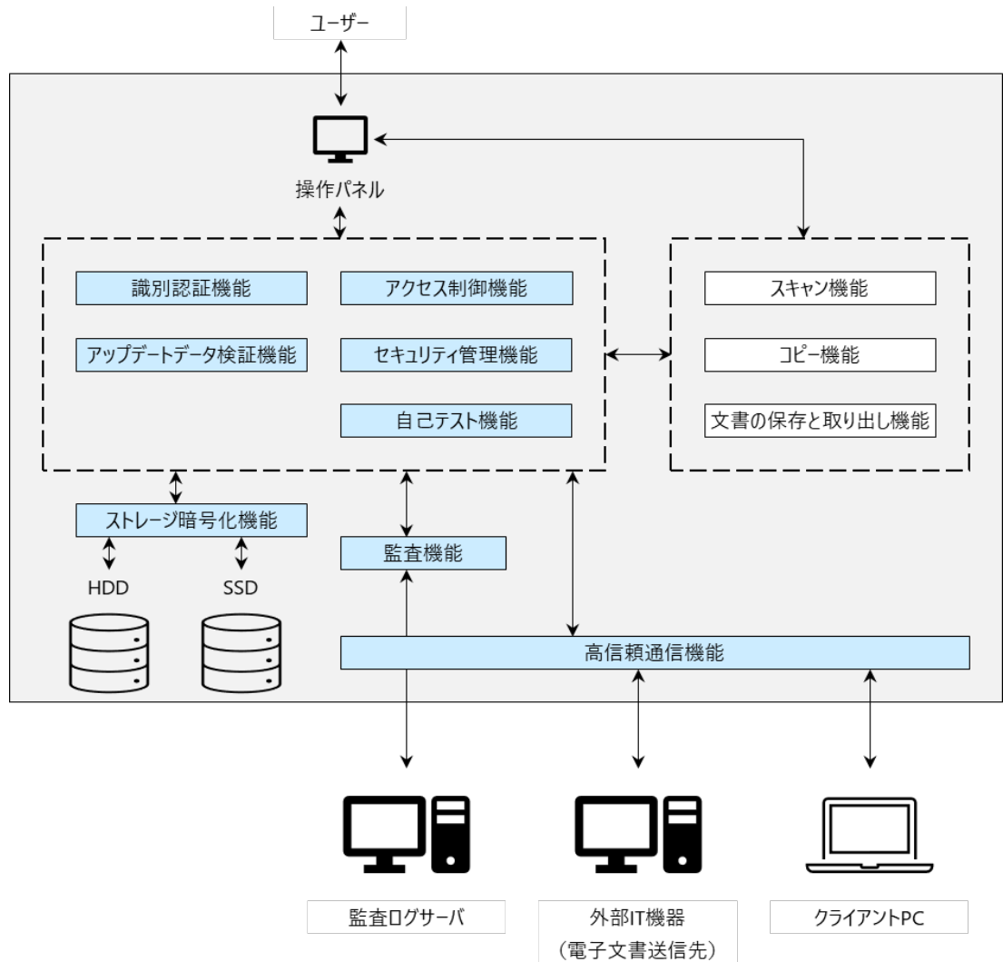
図 5-1 TOE の構成
