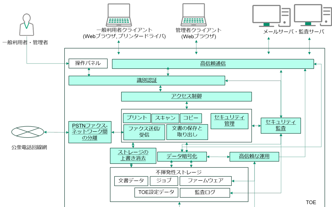
図 2 TOE の論理的構成
