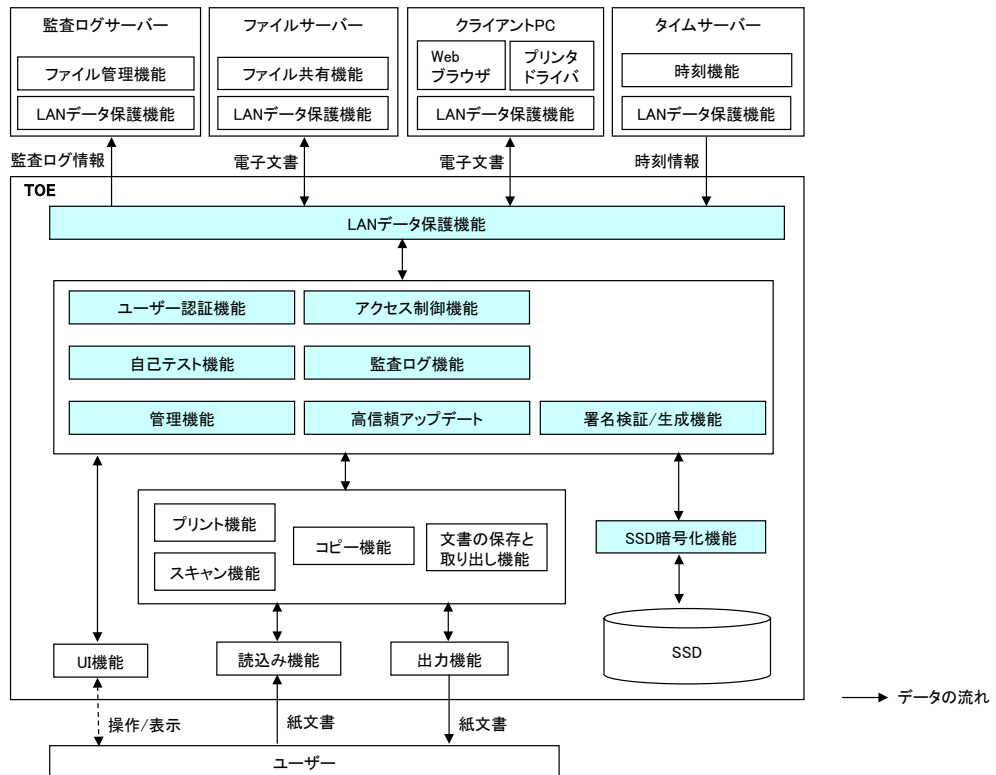
図 5-1 TOE の構成
