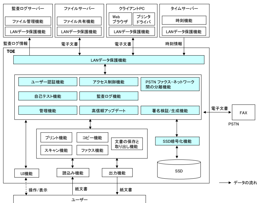
図 5-1 TOE の構成
