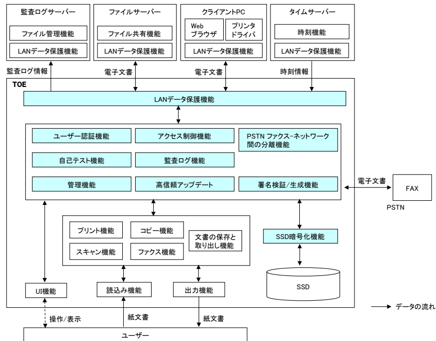
図 5-1 TOE の構成
