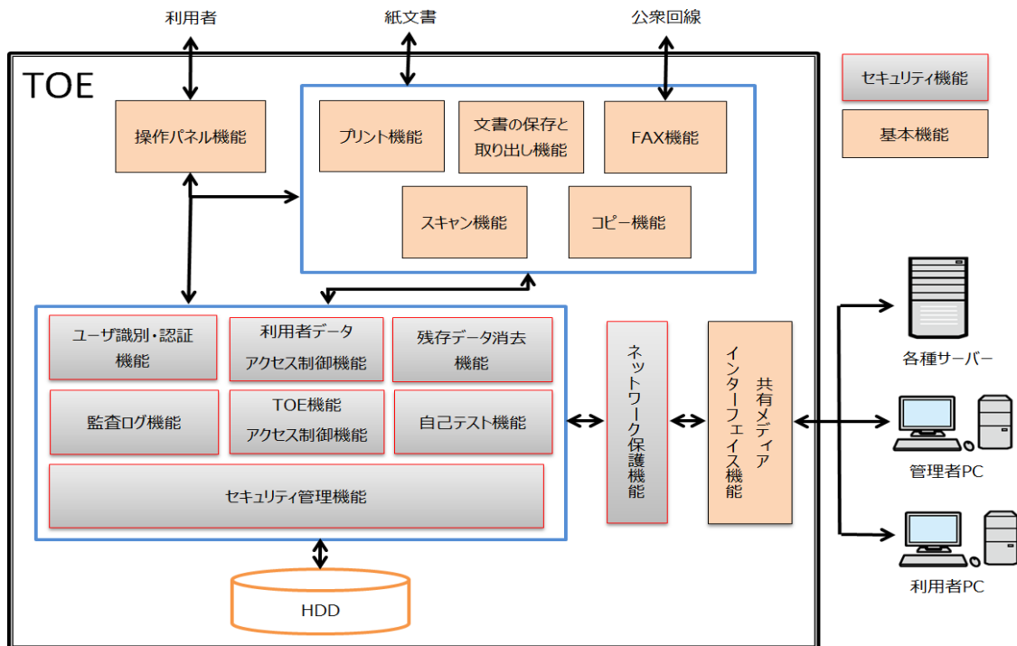
図 1-2. TOE の論理的範囲
