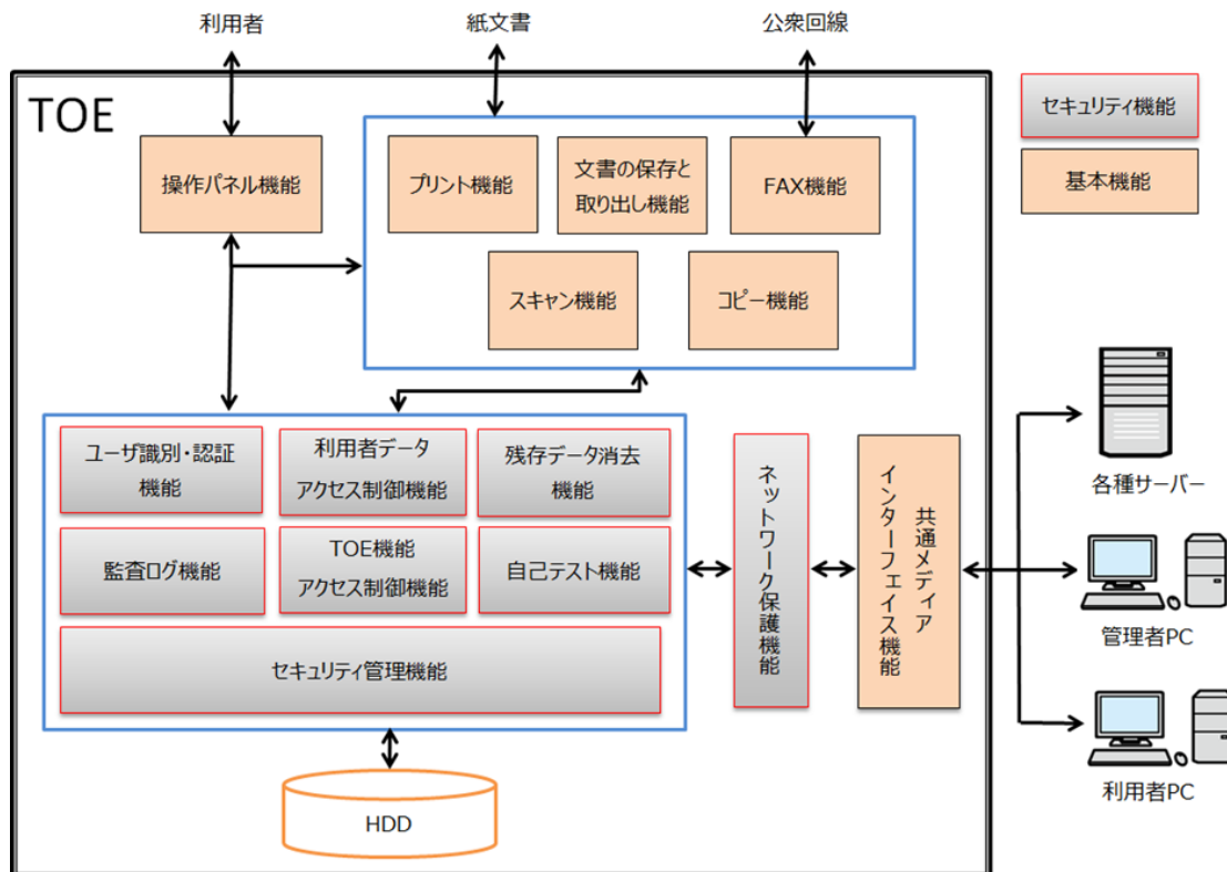
図 5-1 TOEの構成
