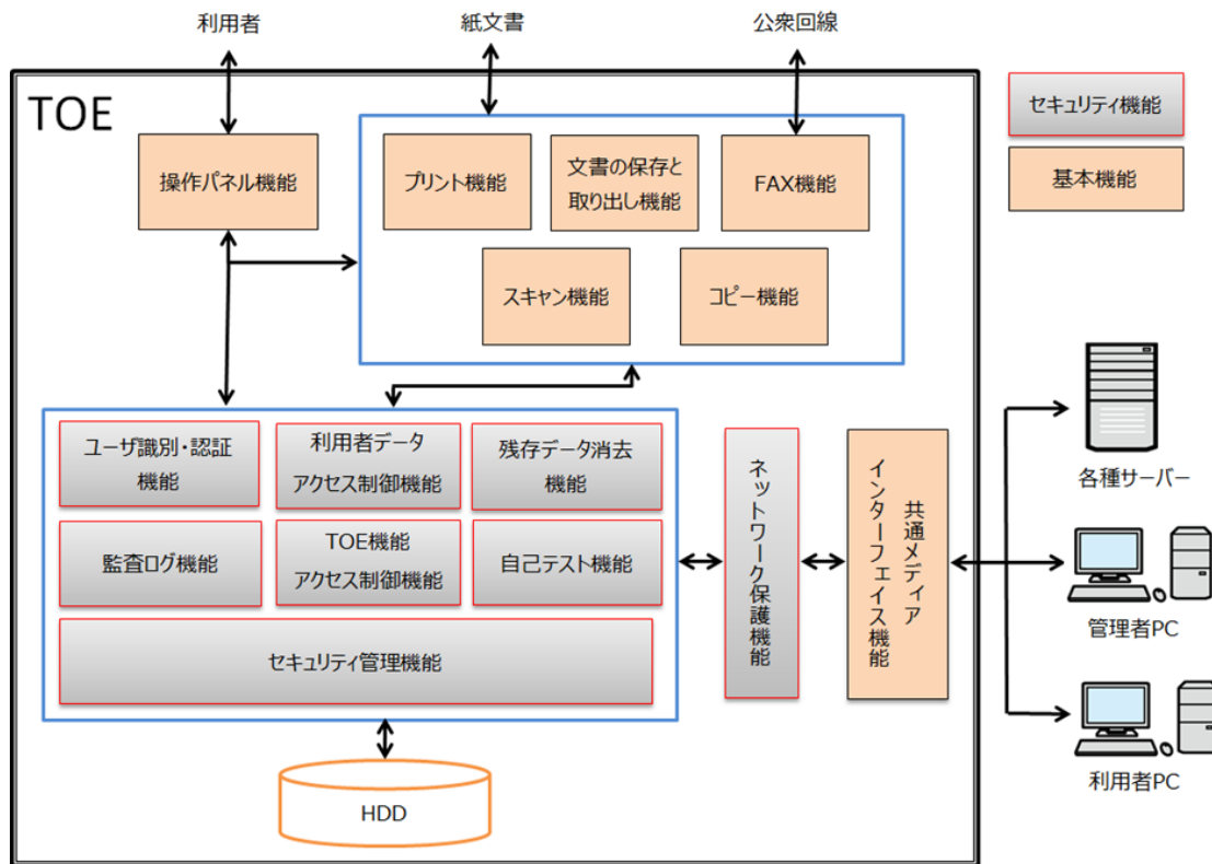
図 5-1 TOEの構成
