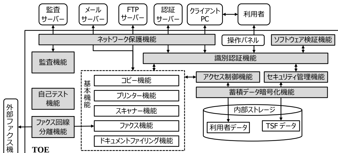
Figure 2: TOE の論理的構成
