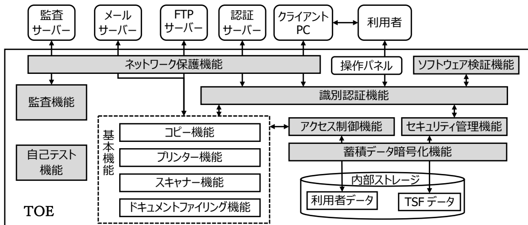
図5-1 TOE 境界
