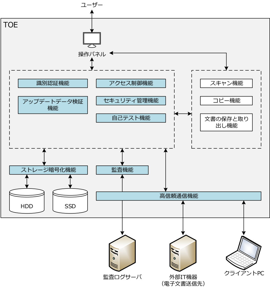
Figure 1-2 TOE の論理的範囲
