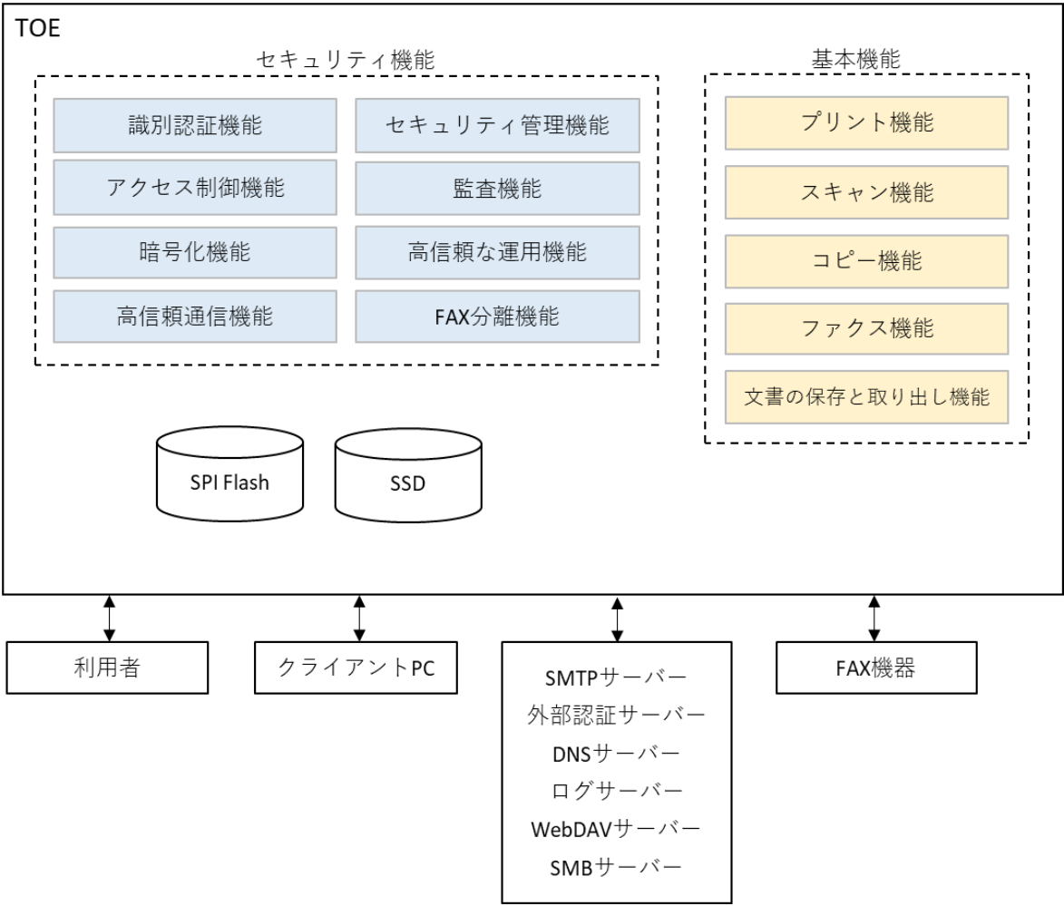
図 5-1 TOE の構成
