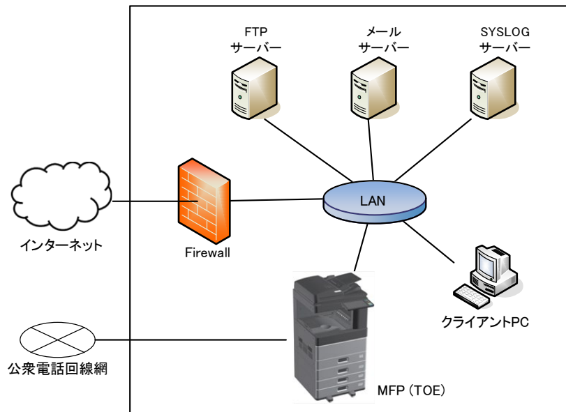
図4-1 TOE の運用環境
