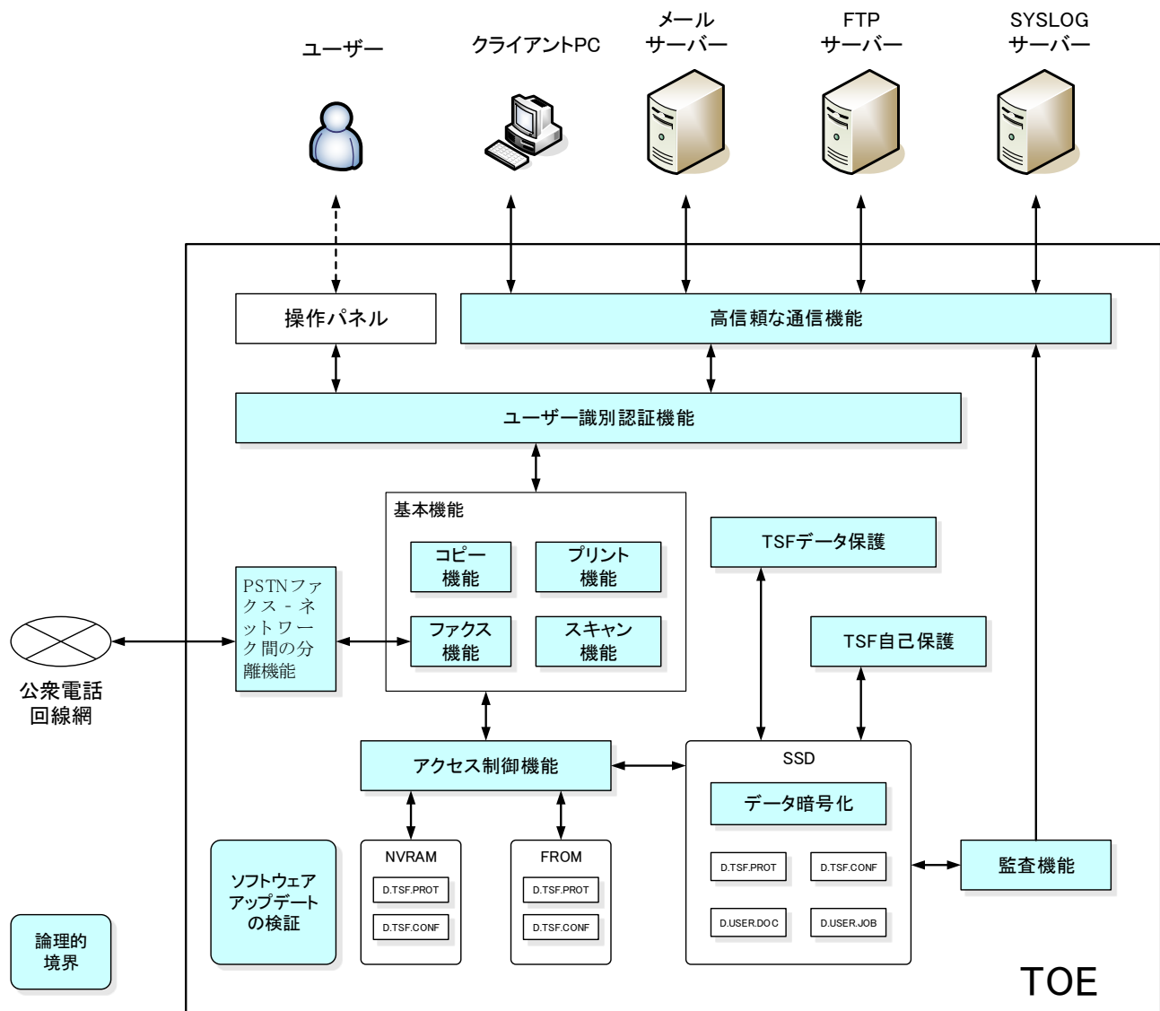
図 2 論理的境界
