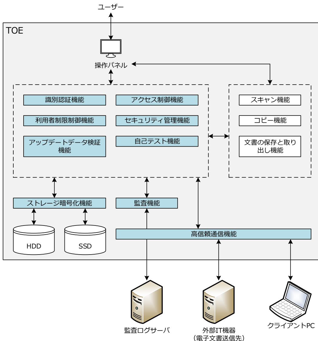
図 5-1 TOE の構成
