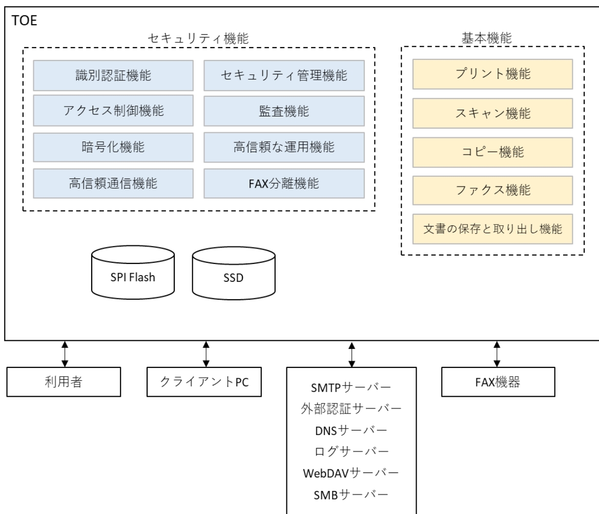
図 5-1 TOE の構成
