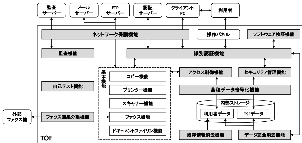
Figure 3: TOE の論理的構成
