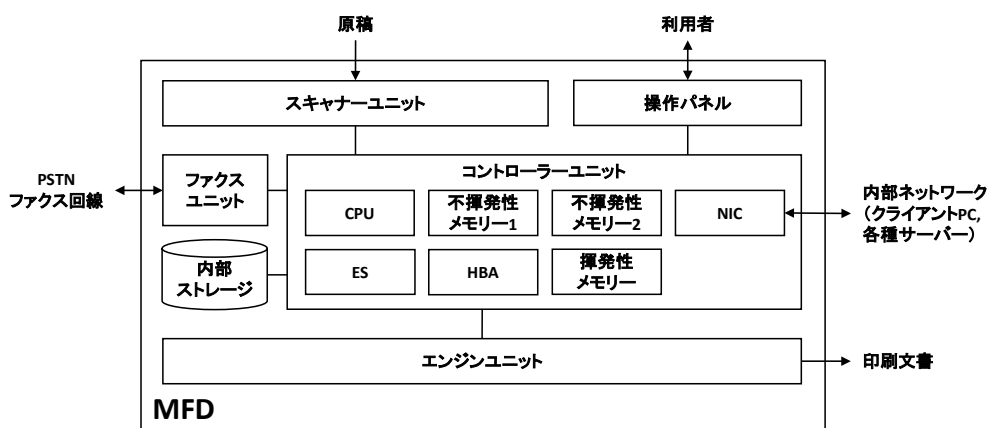
Figure 2: TOE の物理的構成
