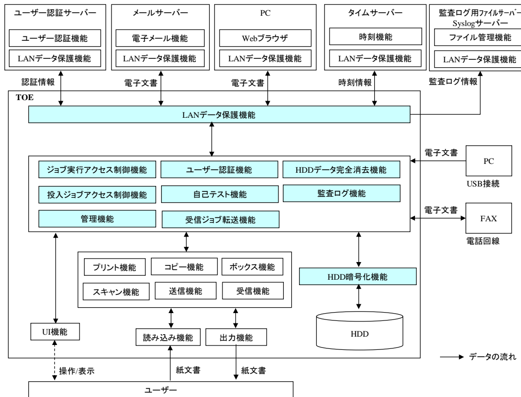
図 5-1 TOE 境界
