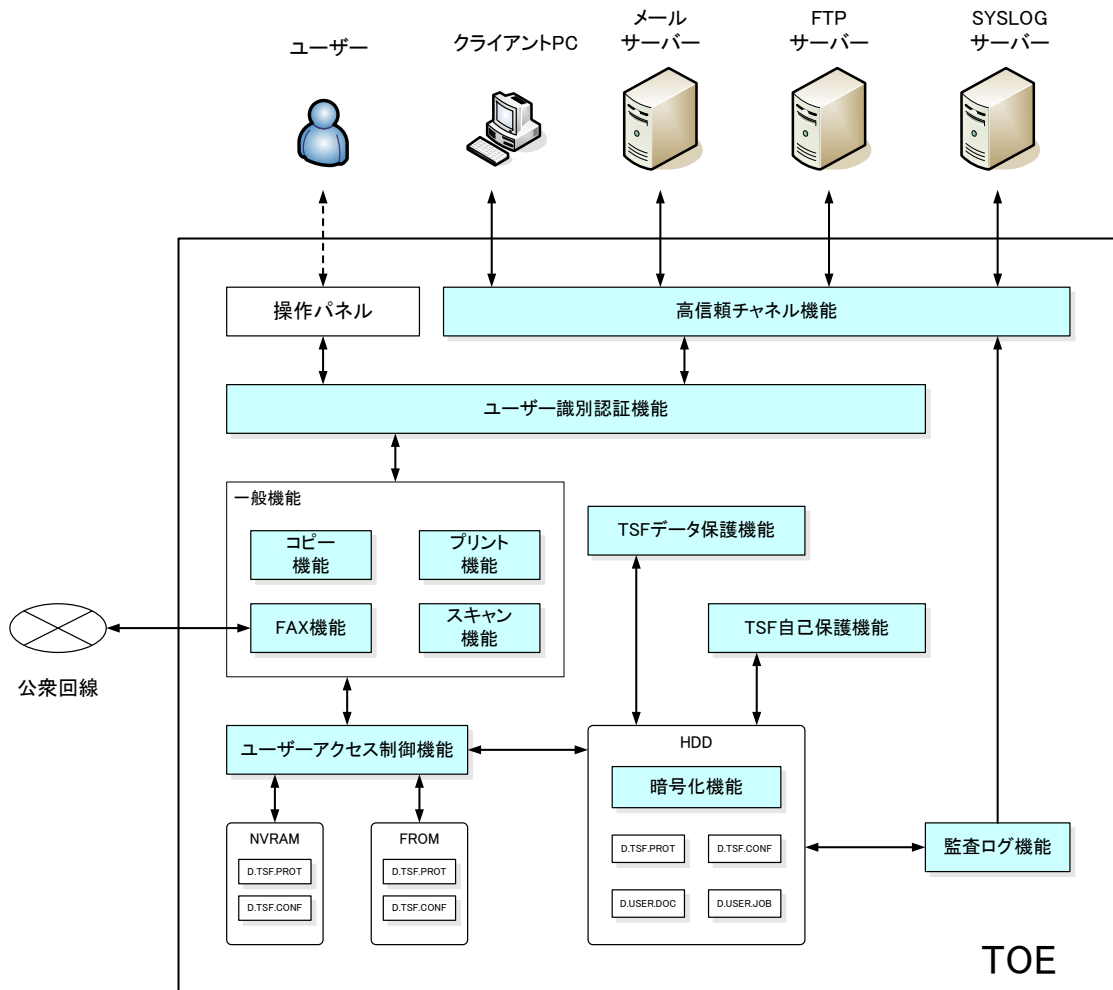
図5-1 TOE境界
