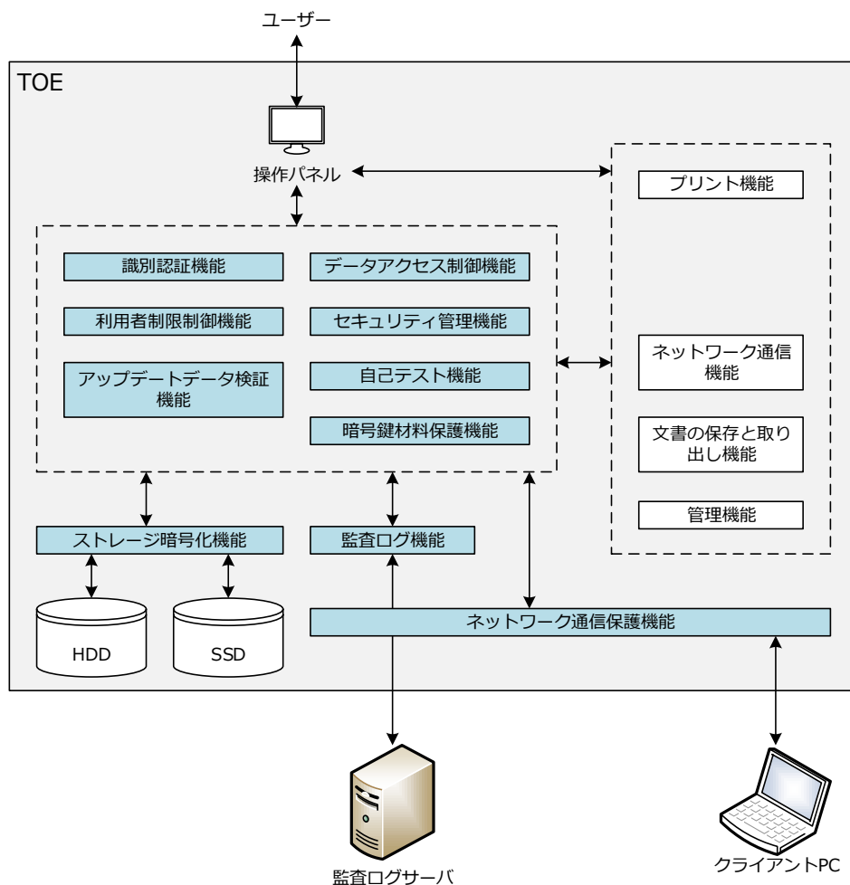
図 5-1 TOE 境界
