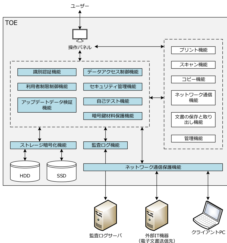
図 5-1 TOE境界
