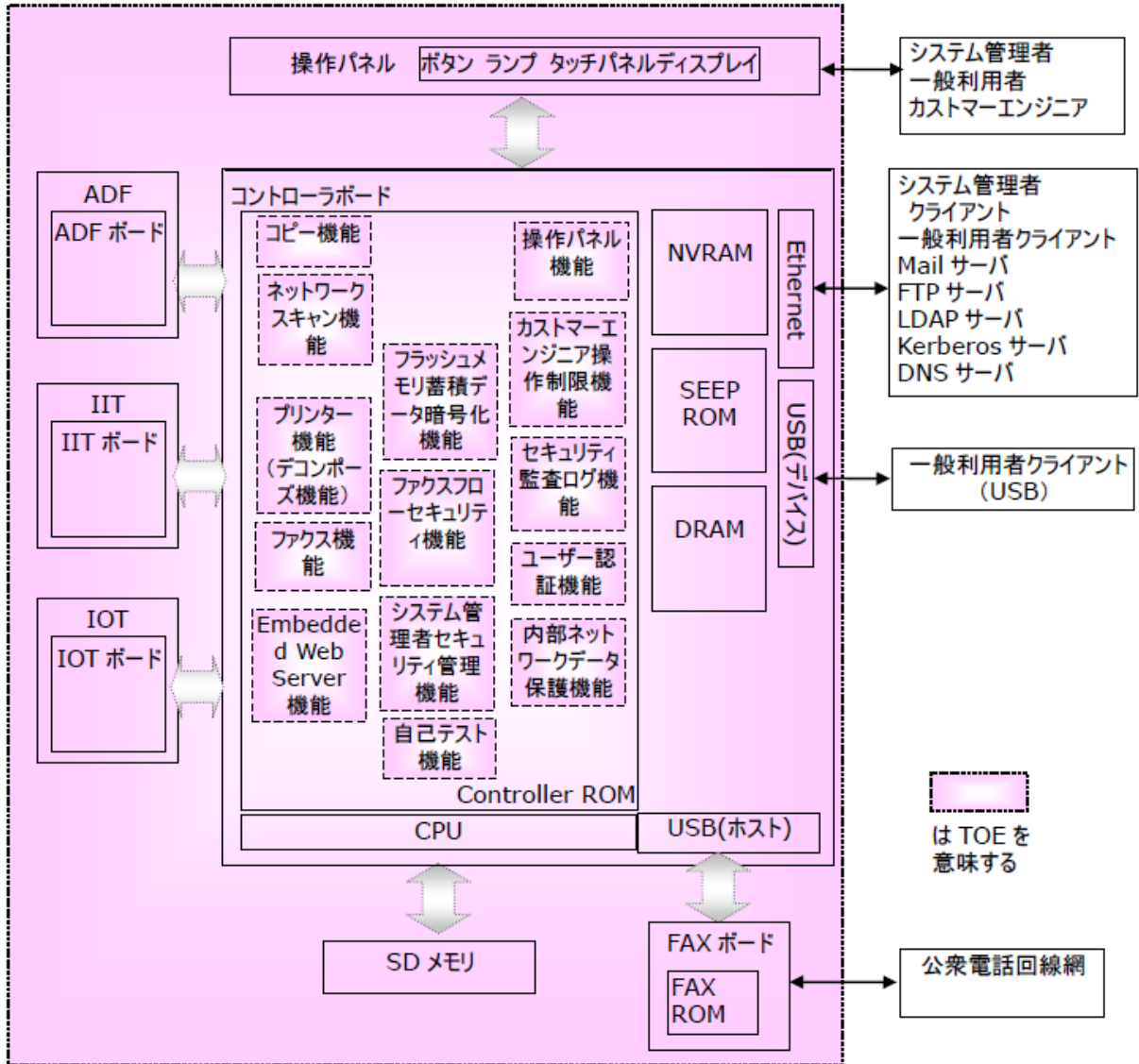
図 5-1 TOE の構成
