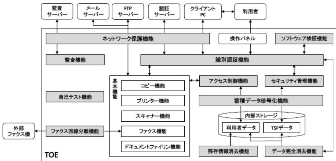
図 5-1 TOE境界
