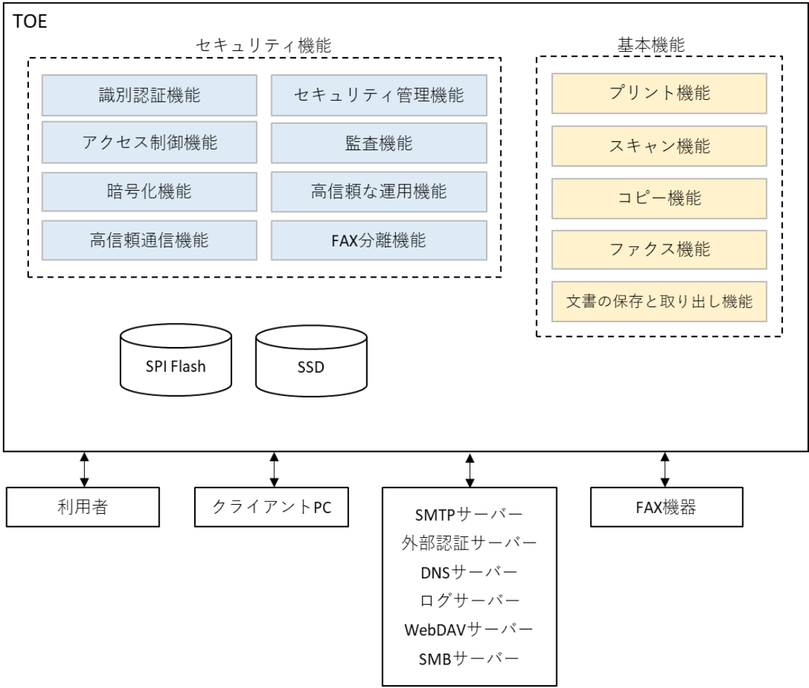
図 5-1 TOE の構成
