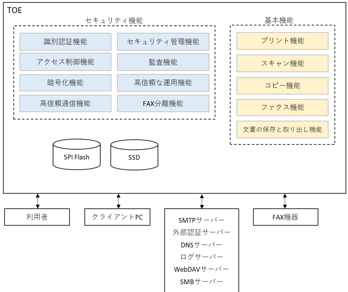
図 5-1 TOE の構成
