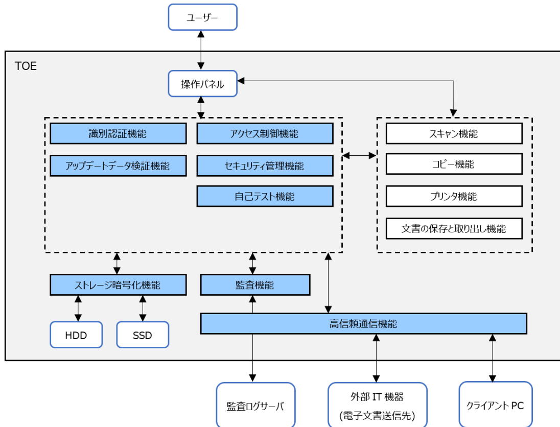
図 5-1 TOE の構成
