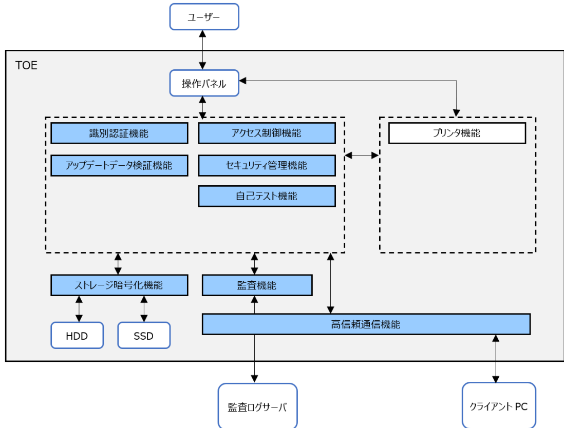
図 5-1 TOE の構成
