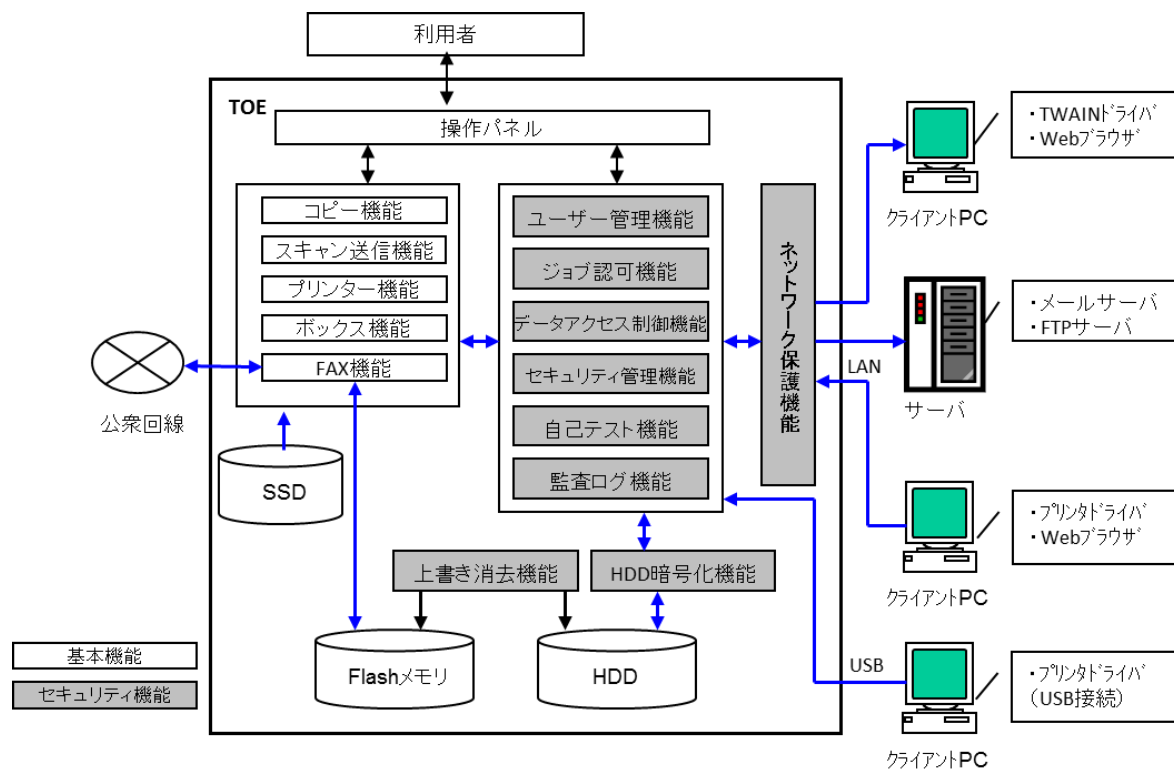
図 5-1 TOE の構成
