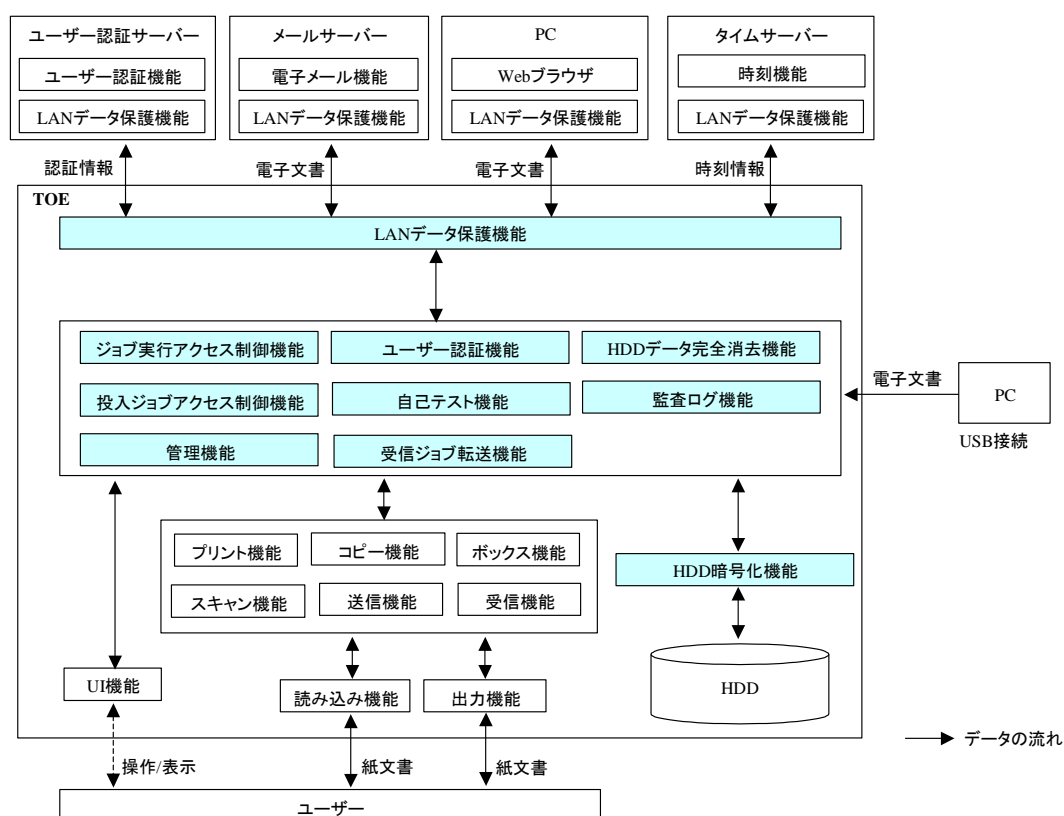
図5-1 TOE境界
