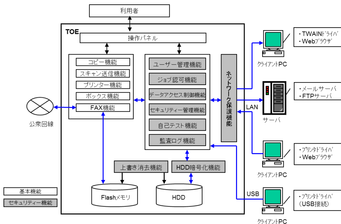
図 5-1 TOE の構成
