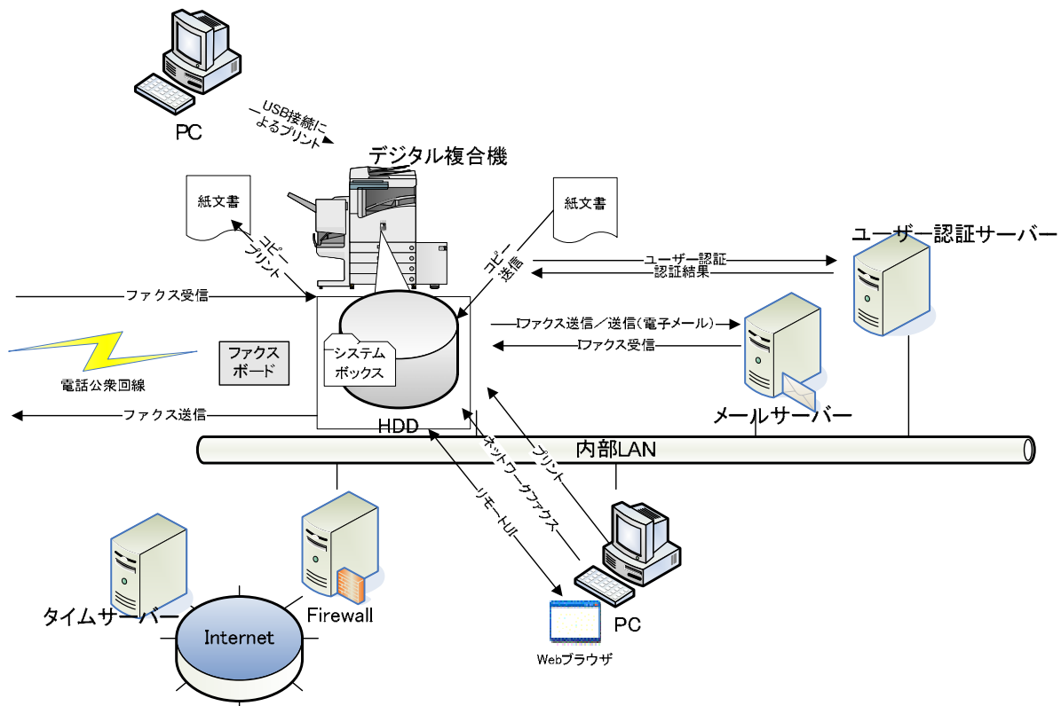
Figure 1 デジタル複合機< Canon imageRUNNER ADVANCE C2200 Series >の想定設置使用環境
