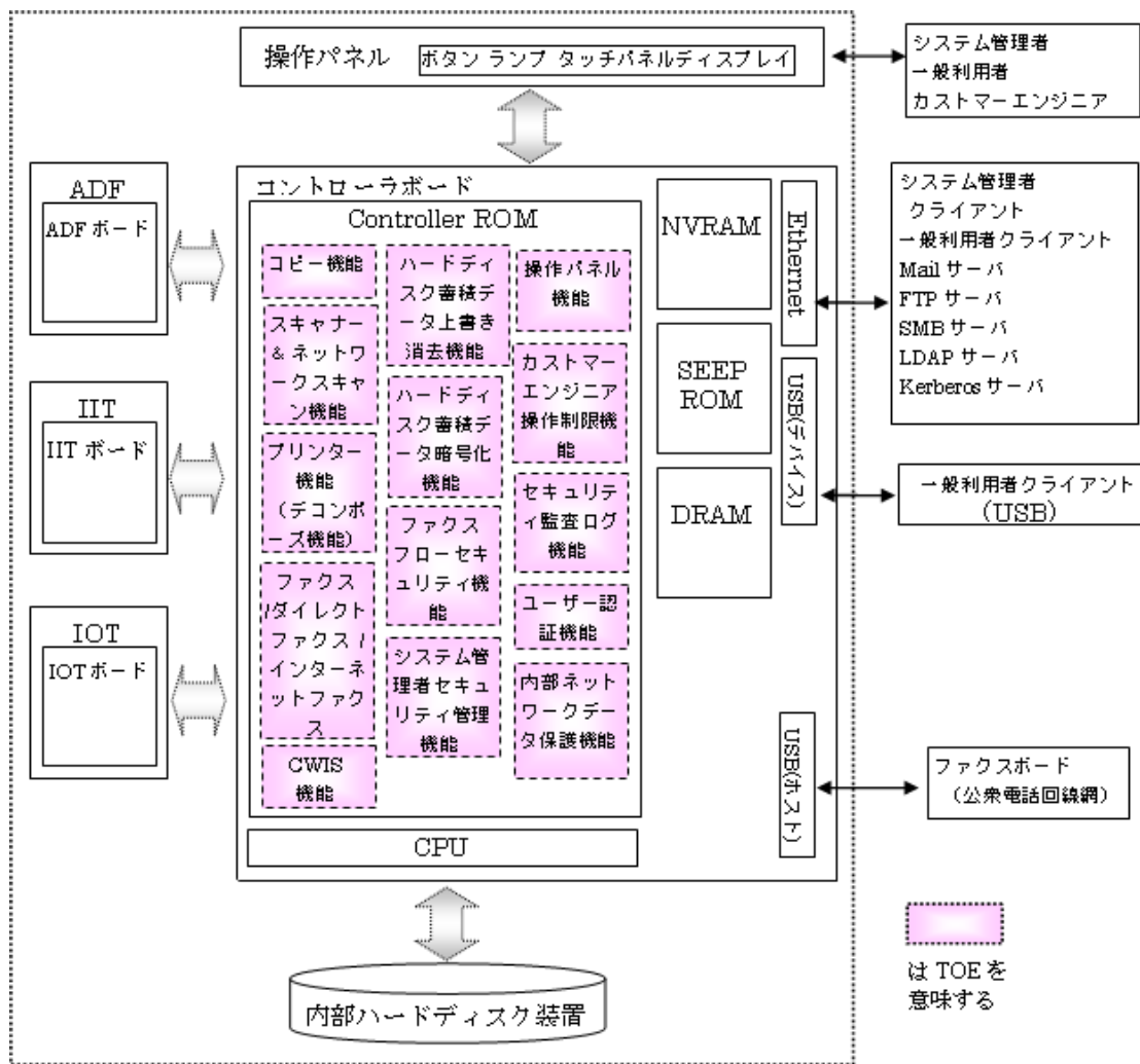
図 5-1 TOE境界
