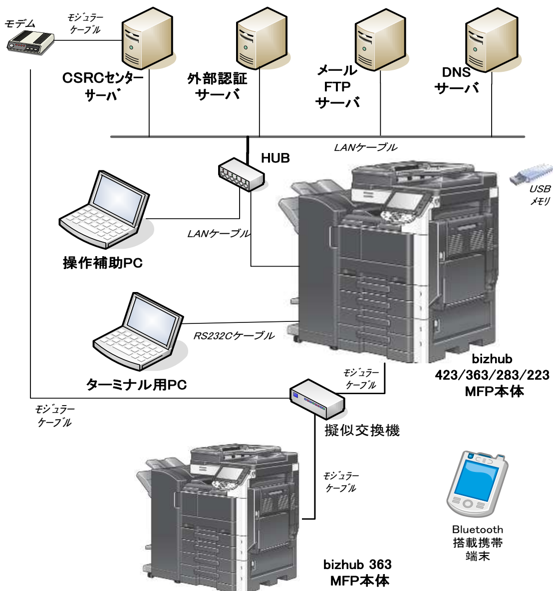
図7-1 開発者テストの構成図
