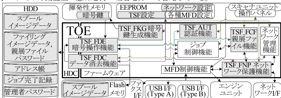
図 3: TOEの論理的構成図
