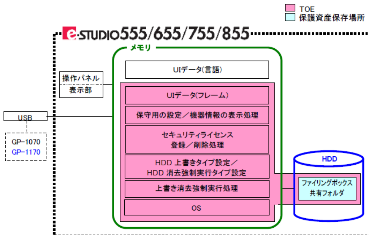
図1-3 自己診断モードの構成
