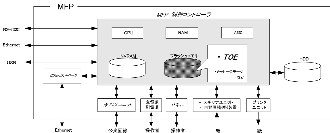
図1-1 TOEに関するハードウェア構成
