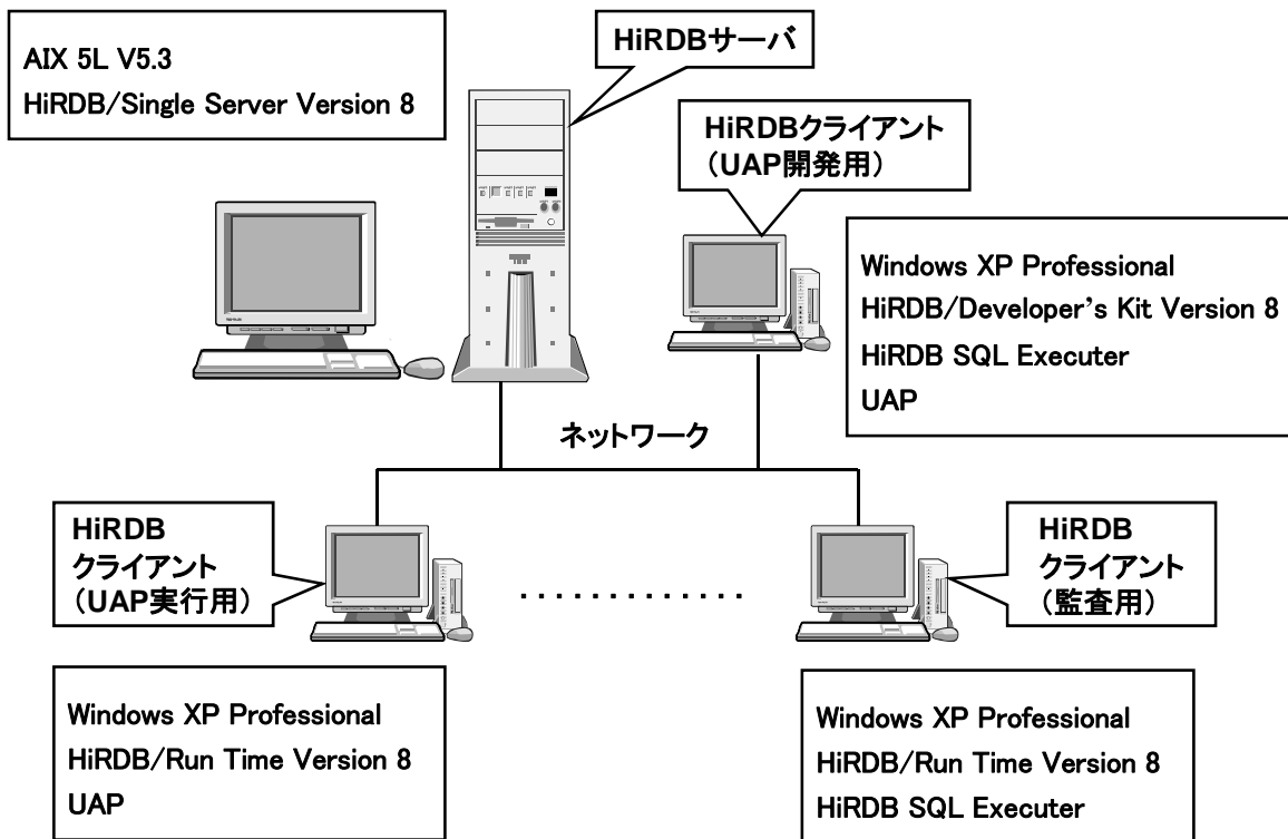
図 2-1 : クライアントーサーバ(C/S)型のシステム構成
