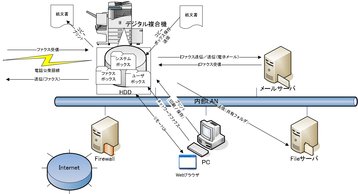
Figure 2-1 デジタル複合機<Canon iR3025/iR3030/iR3035/iR3045 Series>の想定設置使用環境
