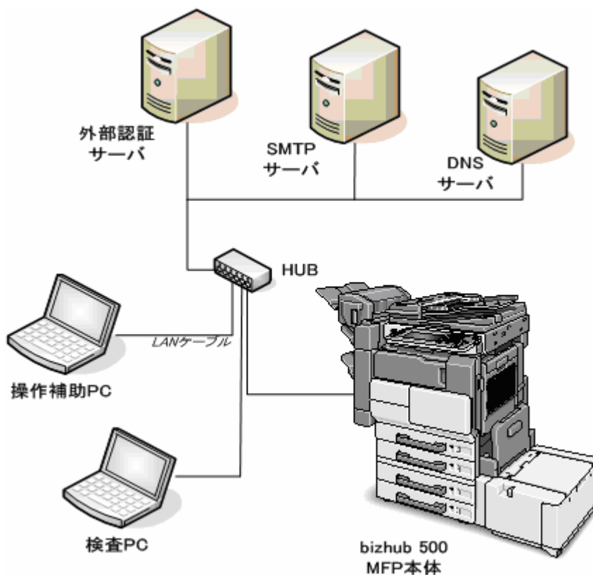
図2-2 評価者テストの構成図
