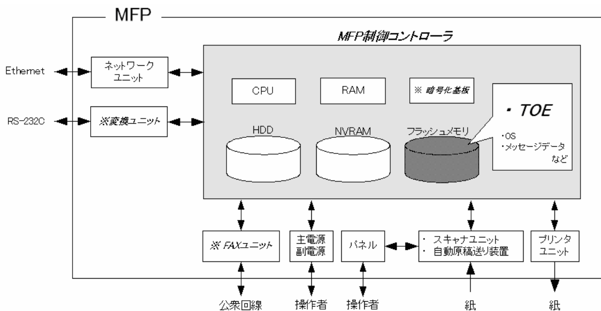
図2-1 開発者テストの構成図
