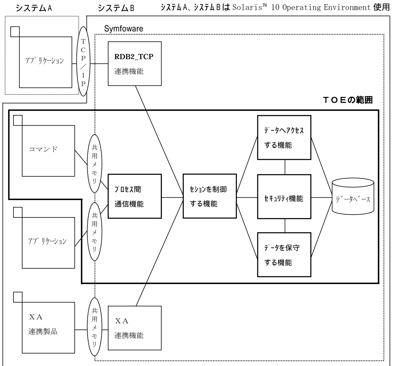
図 2. 2 機能構成
