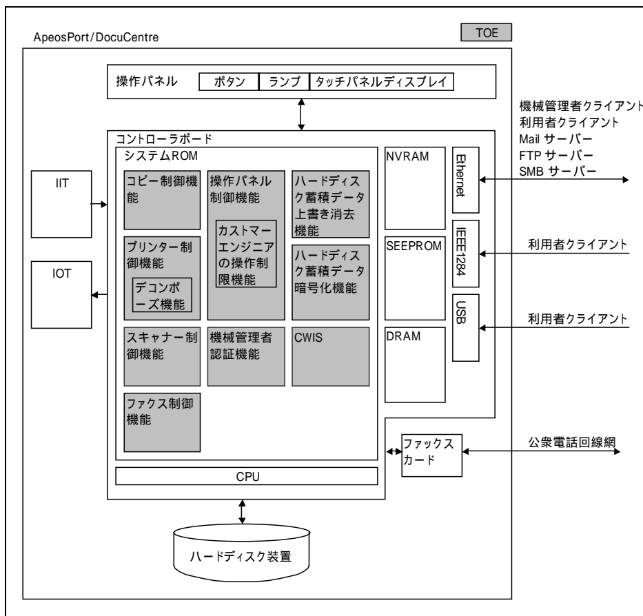
図1-1 TOEの物理的構成イメージ
