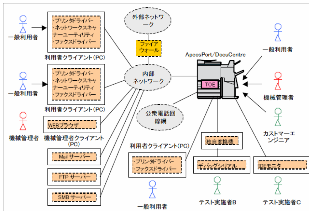
図2-1 開発者テストのシステム構成
