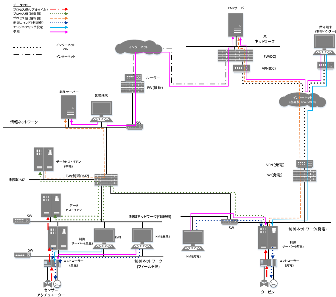
図 2-3 データフロー図(全体)
