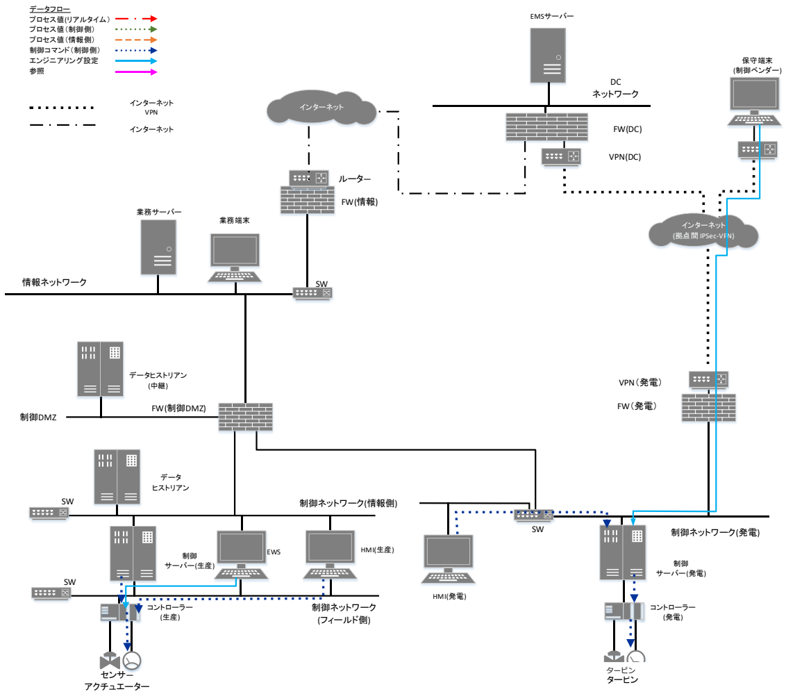
図 2-4 データフロー図(制御・エンジニアリング)
